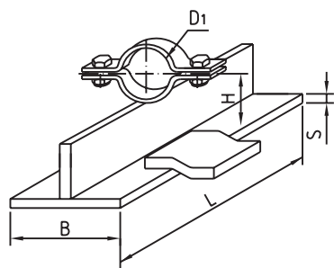
Gleitschellensystem schwer pipe clamp with slide bar heavy
