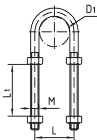
Rohrspannbügel DIN mittel pipe support
