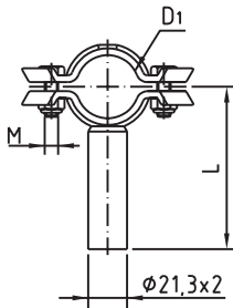
Rohrhalter Zoll, m.Schaft, Typ Skandinavien pipe clamp
