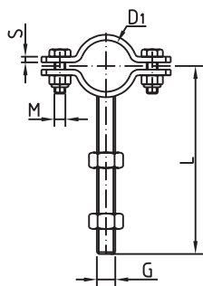
Rohrschelle mit Gewindeschaft pipe clamp with threaded shaft
