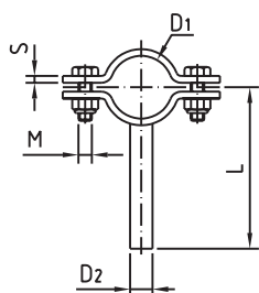
Rohrschelle m. Schaft f. Rohr n. DIN 11850 pipe clamp with welding shaft
