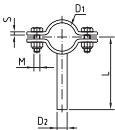
Rohrschelle Zoll, mit Schaft pipe clamp with shaft
