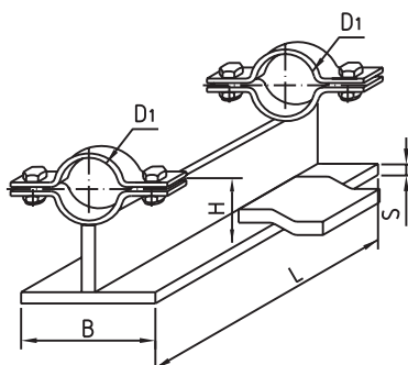
Gleitschellensystem schwer pipe clamp with slide bar heavy
