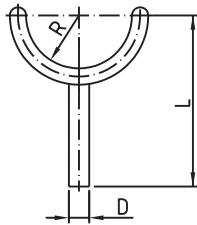
Rohrträger pipe support
