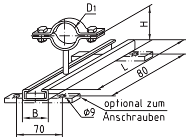
Gleitschellensystem leicht pipe clamp with slide bar light
