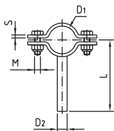
Rohrschelle ISO, leicht, mit Schaft pipe clamp with welding shaft
