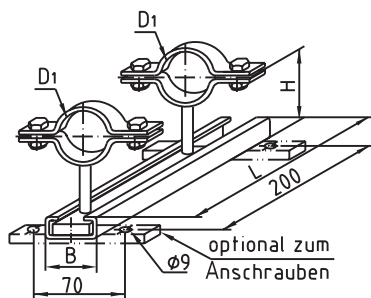
Gleitschellensystem leicht pipe clamp with slide bar light
