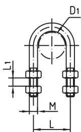
Rohrspannbügel DIN kurz pipe support
