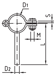
Rohrschelle DIN, klappbar m. Schaft pipe clamp hinged with shaft
